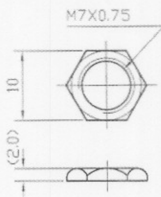
NUT 1PC
